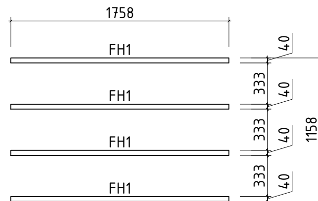
Alustalade plaan / Lagerholzplan / Foundation beams
