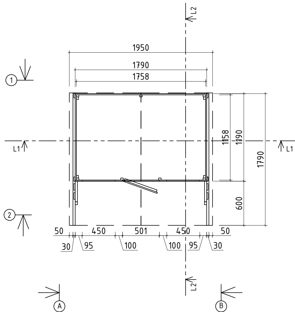
Alustalade plaan / Lagerholzplan / Foundation beams
