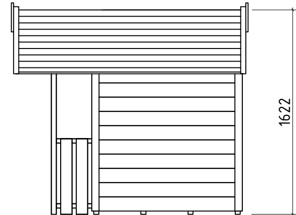
Sein / Wand / Wall B
